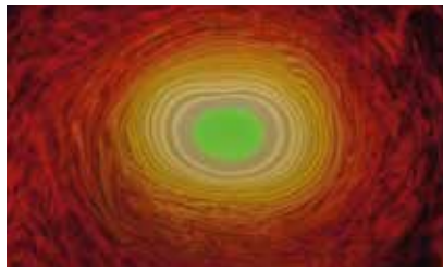
Neutronenstern-Verschmelzung mit Quark-Gluon-Plasma (grün).
